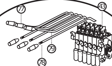
PALANCAS VALVULA COMANDO
