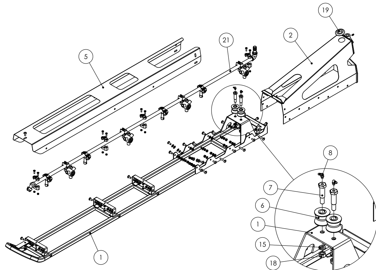
DETALLE B ESCALA 1 : 5
