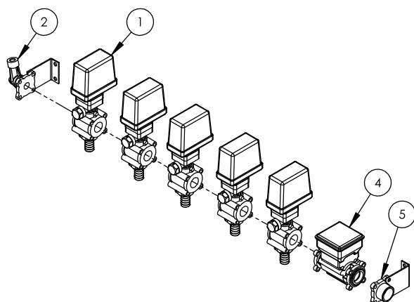
COMANDO SECCIONES MOTRIZ 463CCA01 (cod. 4252)
