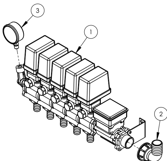
CONJUNTO COMANDO SECCIONES MOTRIZ (cod. 9184)
