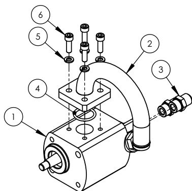
CONJUNTO BOMBA ACEITE HCO.P/DEUTZ - 38 LTS./MIN. - C/TAPA DIV (cod. 14082)
