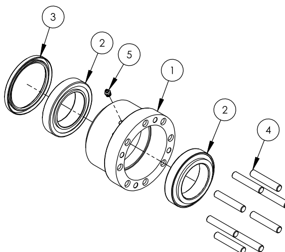
CUBO MAZA FLOTANTE PUNTERA DIFERENCIAL (cod. 2780)
