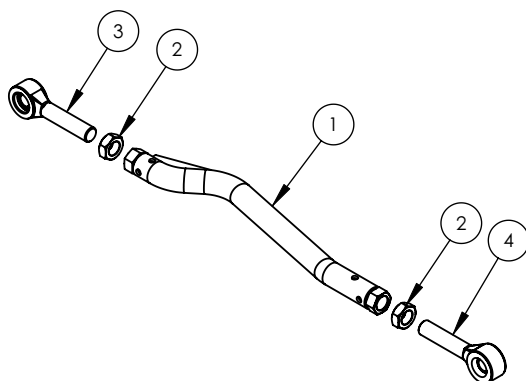
CONJUNTO TENSOR DELANTERO CURVADO (cod. 2832)
