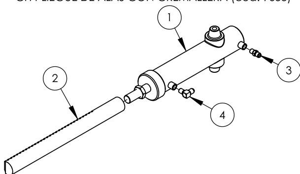
CH PLIEGUE DE ALAS CON CREMALLERA (cod. 9655)
