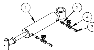
CONJUNTO CH QUIEBRE ALAS (cod. 9552)
