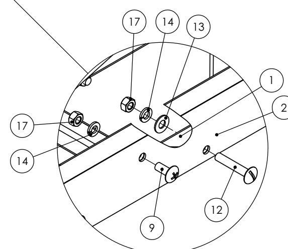
DETALLE E ESCALA 1 : 2.5
