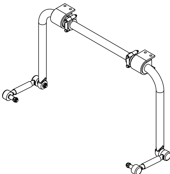
BARRA ESTABILIZADORA DELANTERA C/CONEXIONES COD.11-0410 (cod. 4495)
