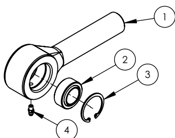
CONJUNTO ROTULA IZQ
