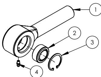
CONJUNTO ROTULA DER
