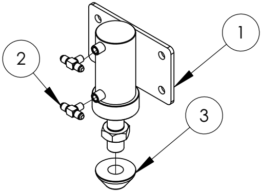
CONJUNTO CH. TRABA BARRAL (cod. 14871)
