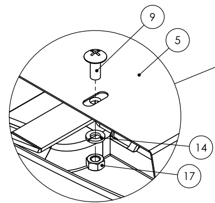
DETALLE C ESCALA 1 : 2
