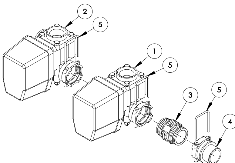
COMANDO CORTE Y REG.MOTRIZ ( 453CCA01 ) (cod. 4209)
