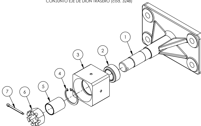
CONJUNTO EJE DE DION TRASERO (cod. 3248)
