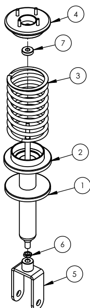
CONJUNTO RESORTE AMORTIGUADOR BOTALÓN (cod. 3033)
