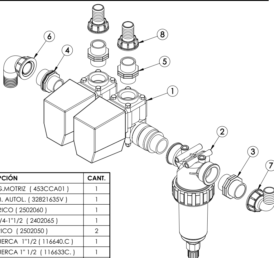
COMANDO CORTE Y REG.MOTRIZ ( 453CCA01 ) (cod. 4209)
