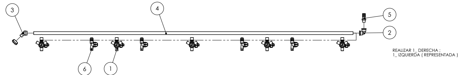
LINEA PUNTERA - 28 - .35/.525 - ZAFE Y (cod. 14540)
