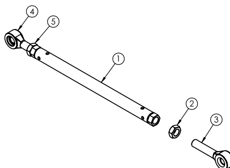
TENSOR DE SUSPENSIÓN DELANTERO (cod. 2934)
