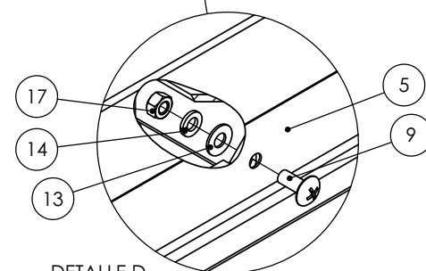
DETALLE D ESCALA 1 : 2.5
