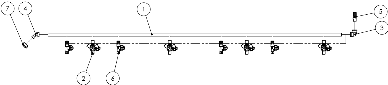
LINEA ALA PUNTERA - 25 - .35/.525 - ZAFE Y (cod. 14275)
