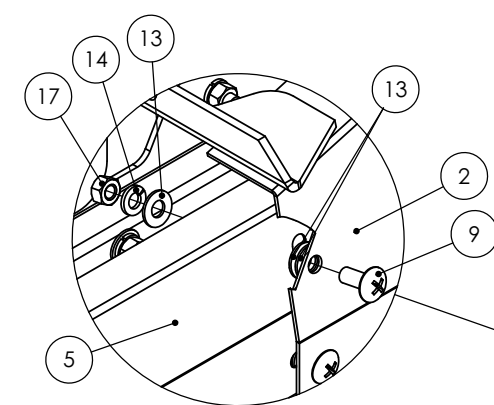
DETALLE J ESCALA 1 : 2.5
