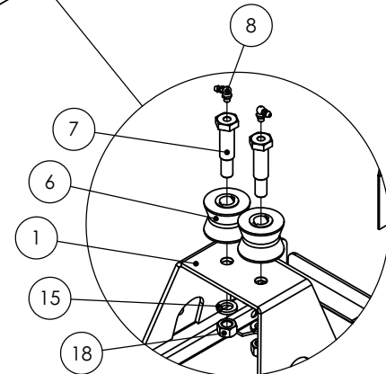
DETALLE B ESCALA 1 : 5
