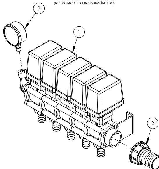
CONJUNTO COMANDO 5 SECCIONES 473 (cod. 16491) (NUEVO MODELO SIN CAUDALÍMETRO)
