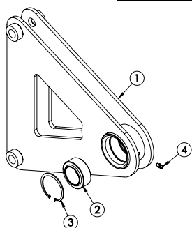
CONJUNTO RESORTE AMORTIGUADOR BOTALÓN (cod. 3033)
