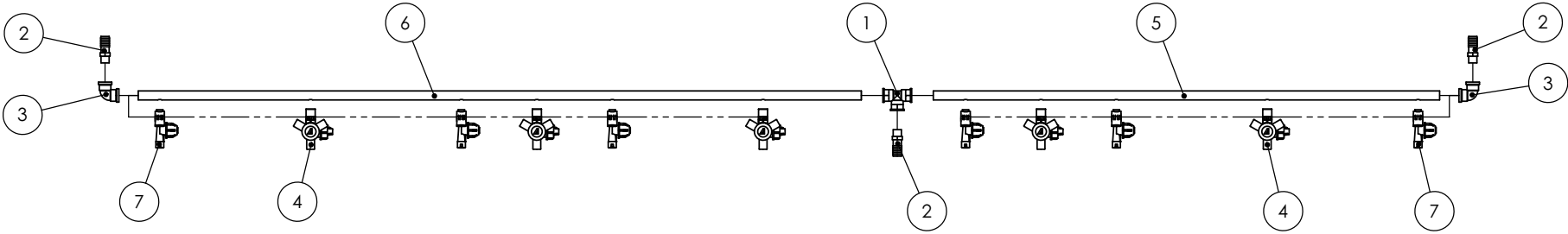
LINEA CENTRAL - 25/28 - .35/.525 (cod. 9163)
