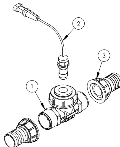
CONJUNTO RAPID-CHECK RM 1 1/2" (cod. 16492)
