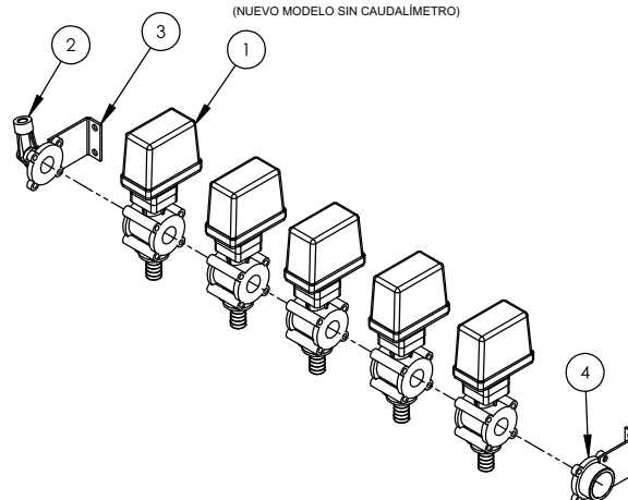
COMANDO SECCIONES MOTRIZ 473CCA01 (cod. 16485) (NUEVO MODELO SIN CAUDALÍMETRO)
