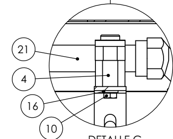
DETALLE G ESCALA 1 : 2
