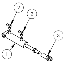
CONJUNTO CILINDRO HIDRÁULICO TRABA BARRAL DE TRANSPORTE (cod. 9557)
