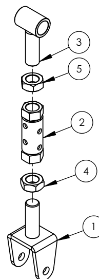
BRAZO SOPORTE CUADRANTE SUSPENDIDO (cod. 3260)
