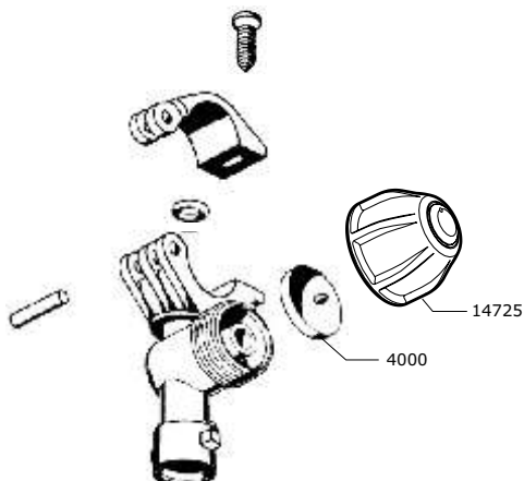
PICO UNIJET HP 1-4 VUELTA 1-2 F10 (COD. 4169)
